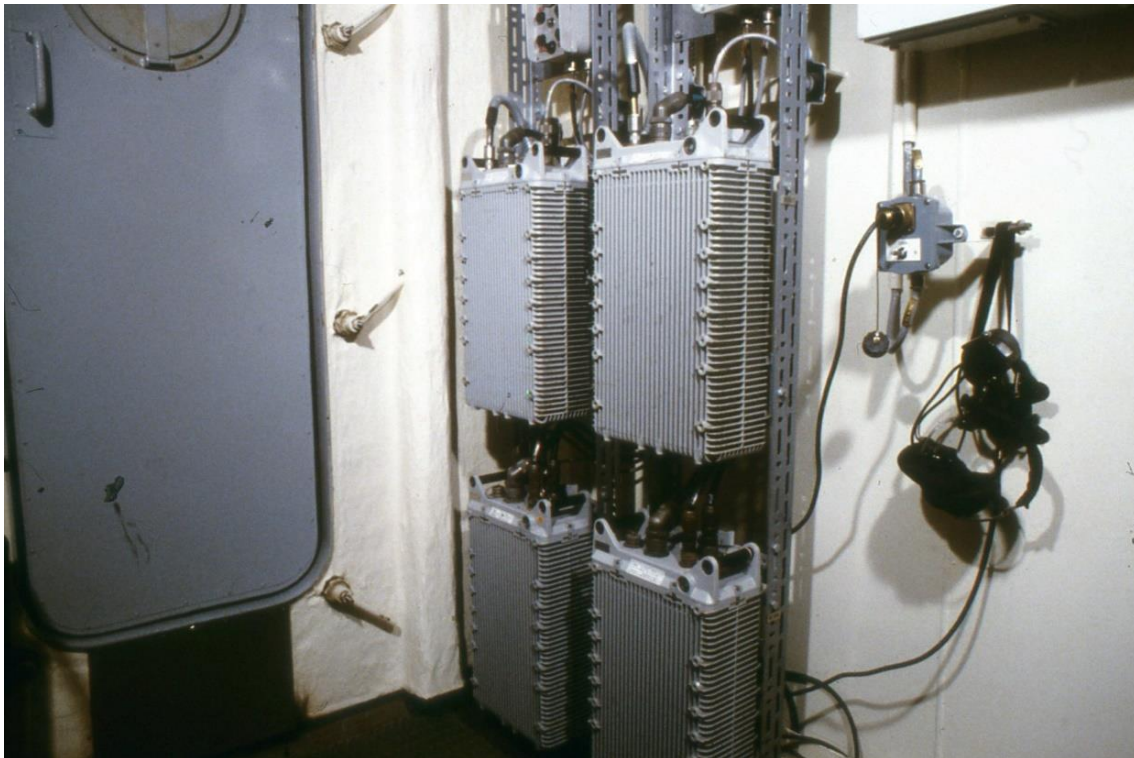
73. Minfartyg typ Carlskrona. Radiohytt C, RA 800
