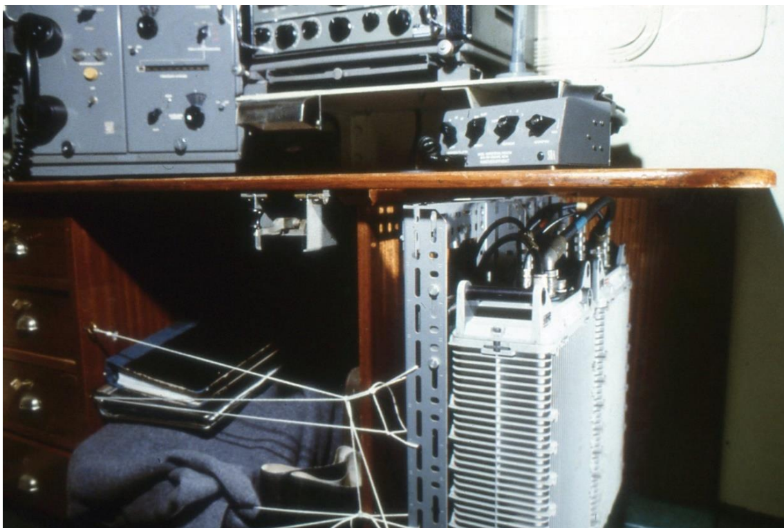
98. Trängfartyg, bogserbåt. Ajax, RA 800 i radiohytt
