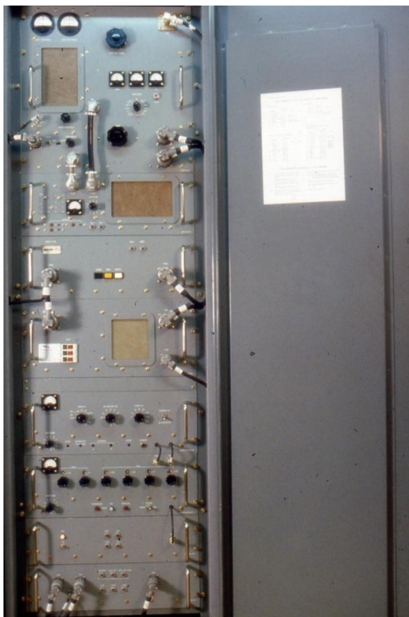
140. Kortvågssändare 763, närbild.
