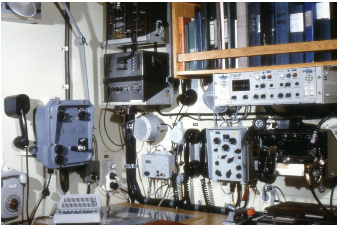
54. Minfartyg typ Älvsborg. Radiohytt A, UK-plats
