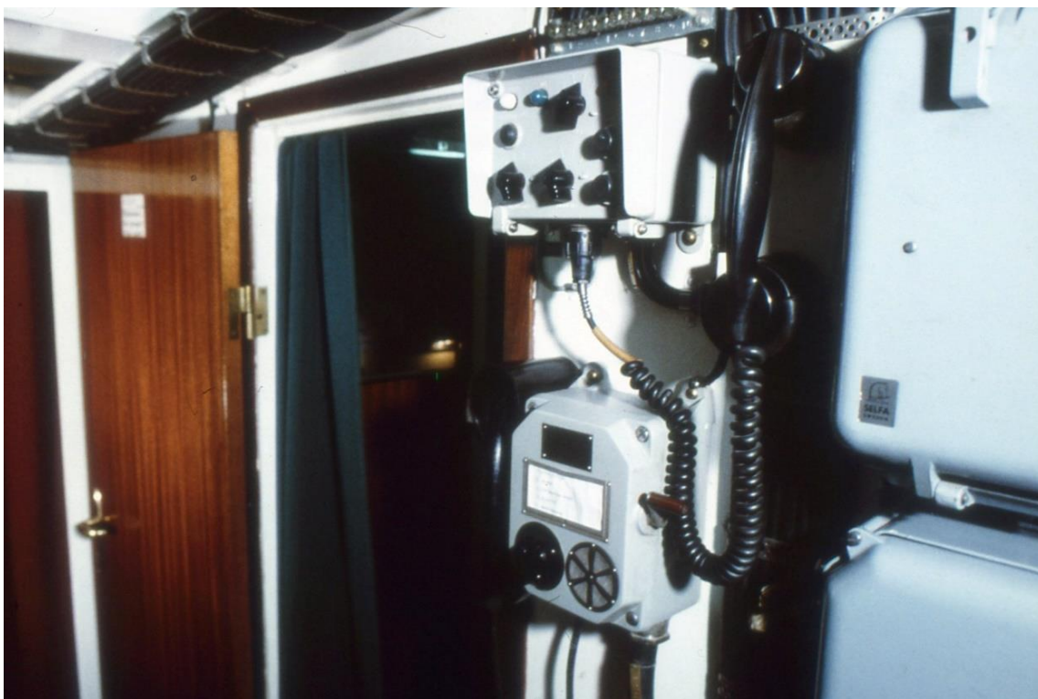
87. Minsvepare typ fiske. Trafikbox RA 800 i gång i bostadsinredning
