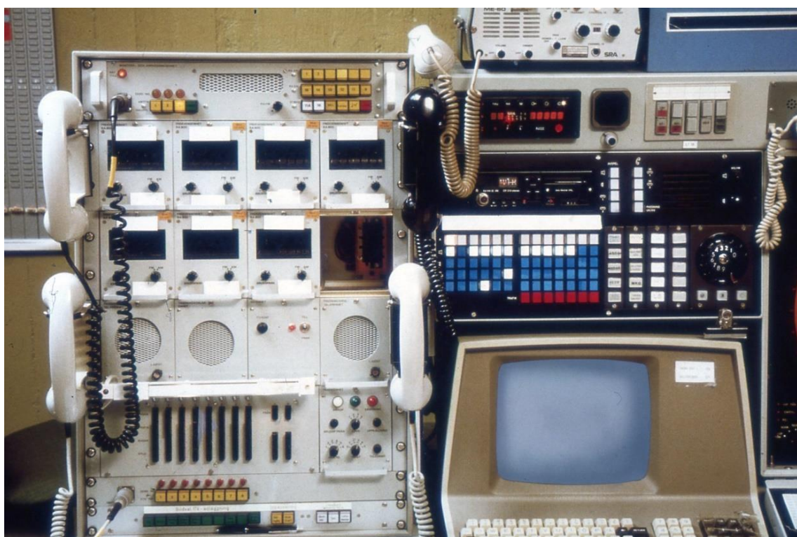
114. Sjöbevakningscentral. Sambandspanel
