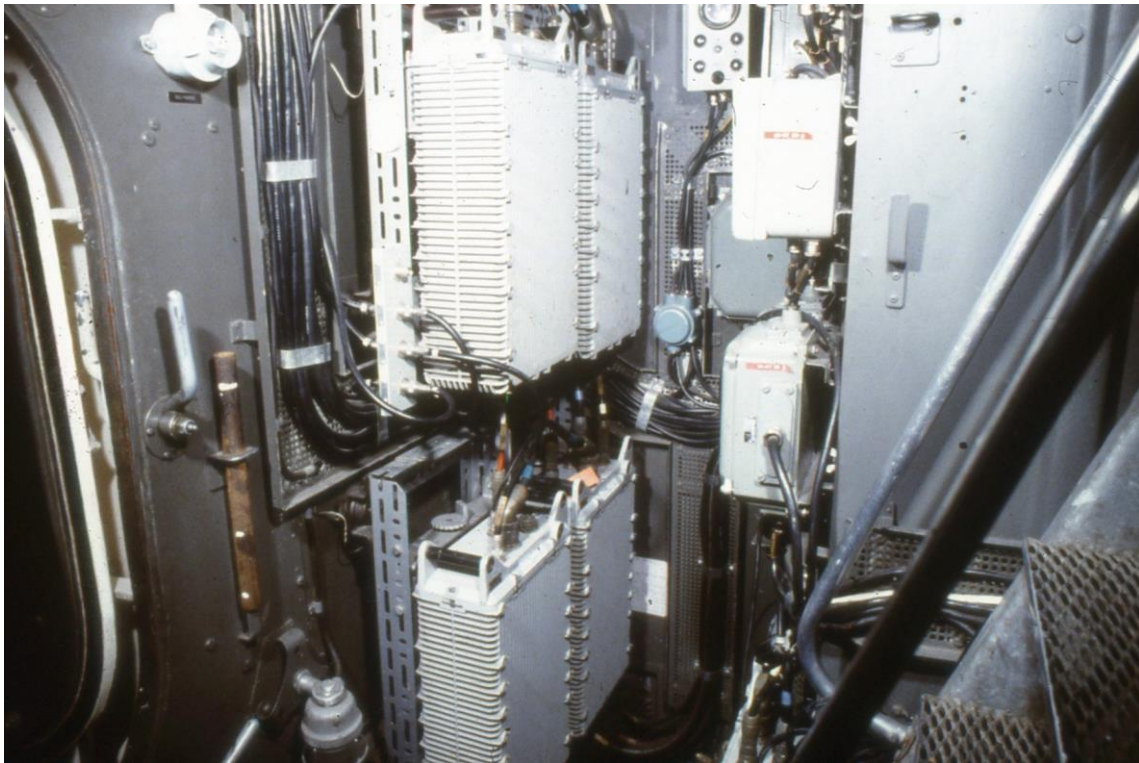
33. Tb typ Spica. Ra 800 i gång utanför stridsledningscentral
