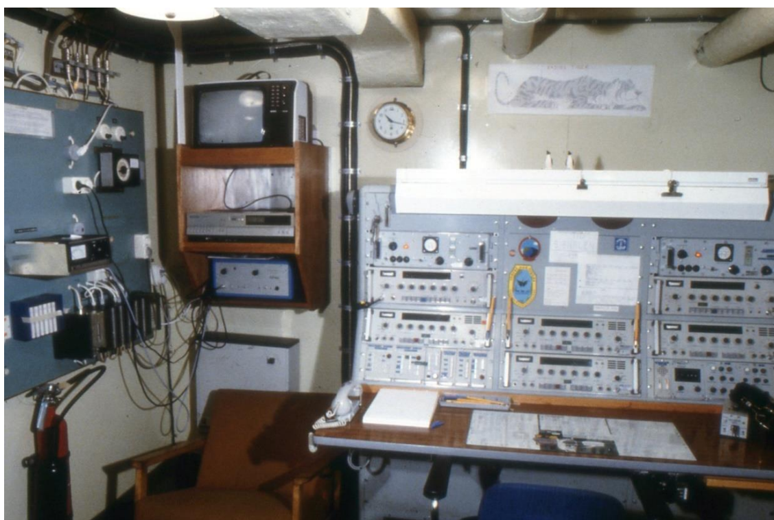
52. Minfartyg typ Älvsborg. Radiohytt A, översikt
