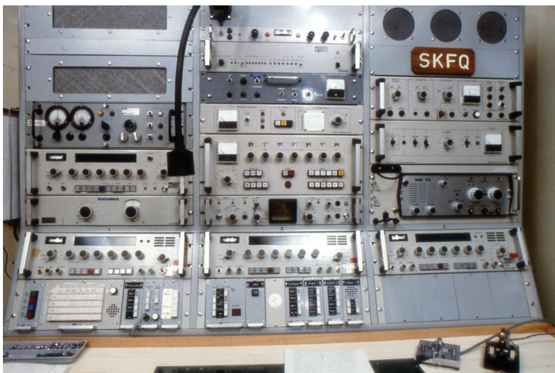
68. Minfartyg typ Carlskrona. Radiohytt A, huvudstativ
