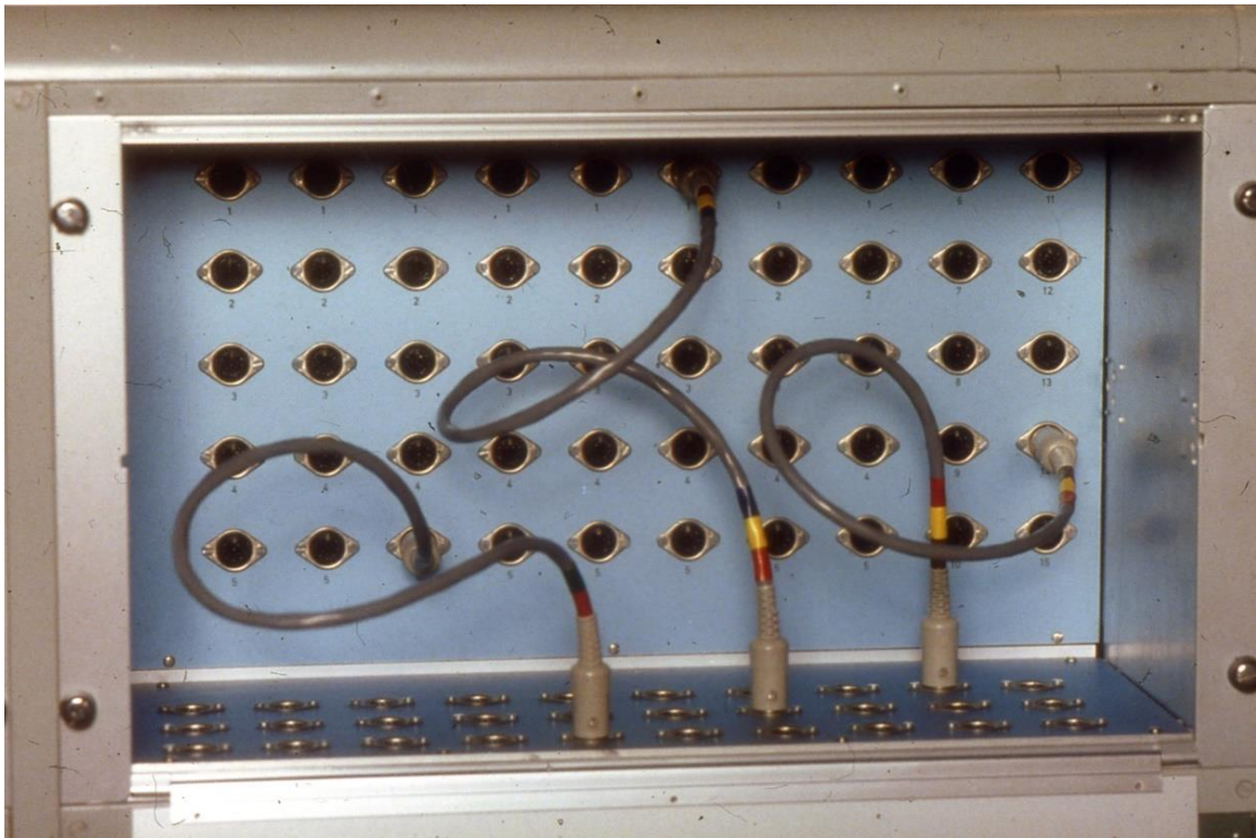
105. Linjefält i modifierad order- rapportkopplare m/51
