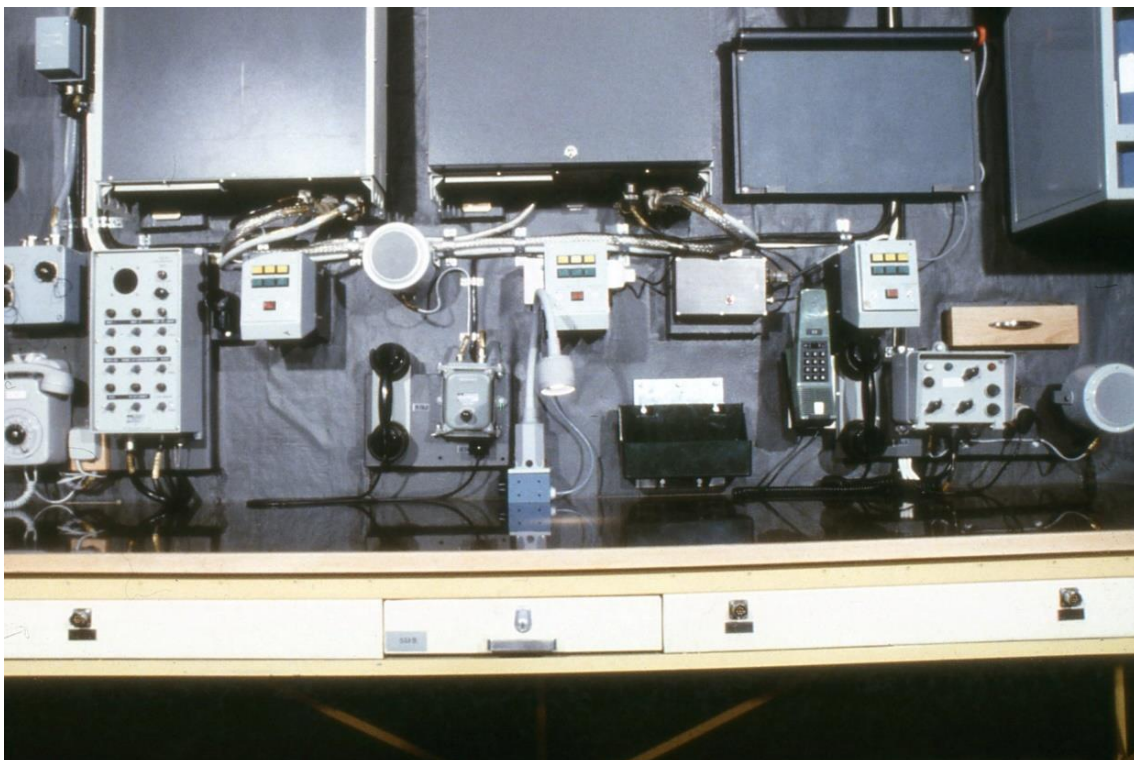
74. Minfartyg typ Carlskrona. Stridsledningscentral, UK-plats
