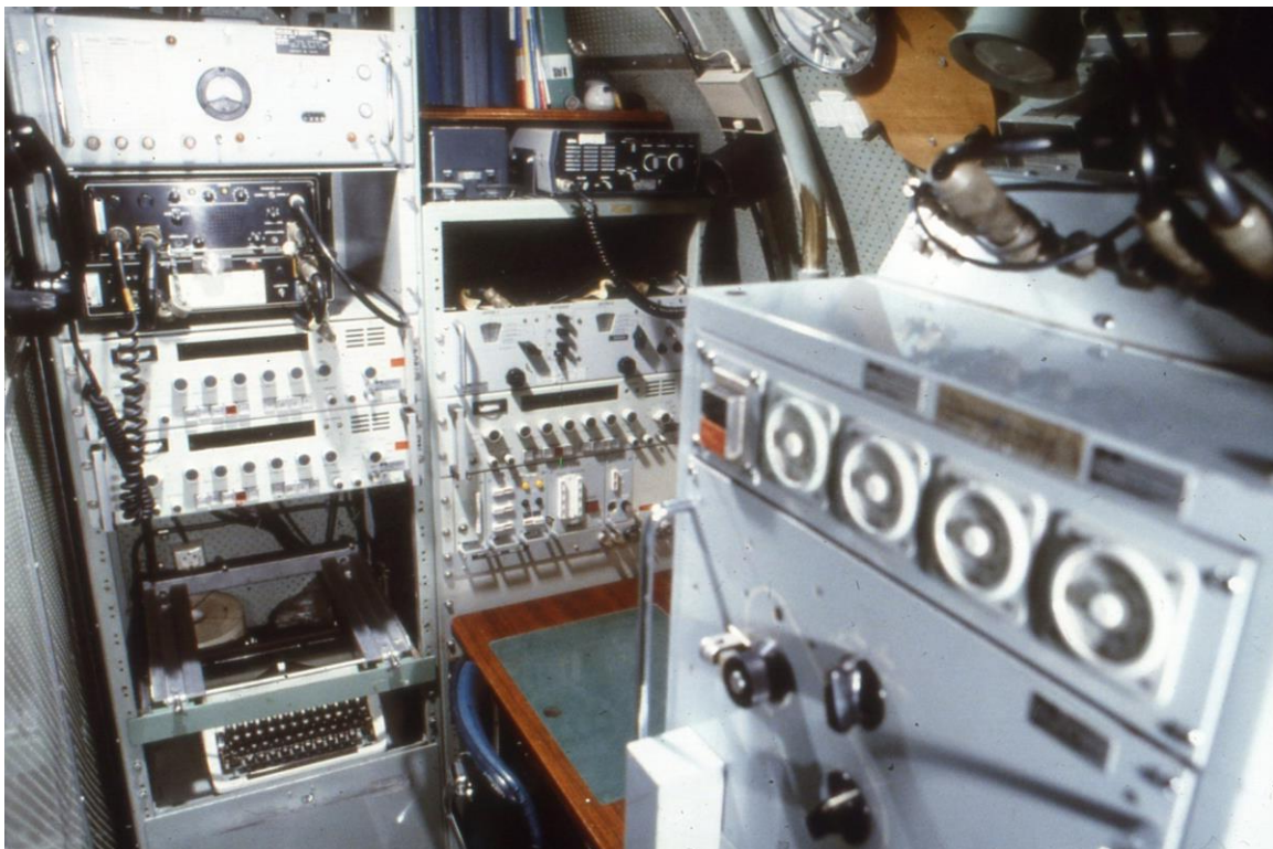
4. Ub typ Draken. Radiohytt, betjäningsplats
