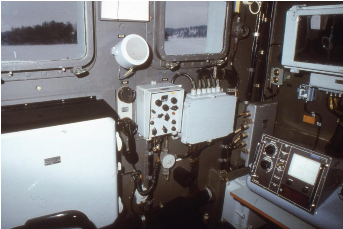
79. Minsvepare typ kust. Styrhytt, styrbords sida
