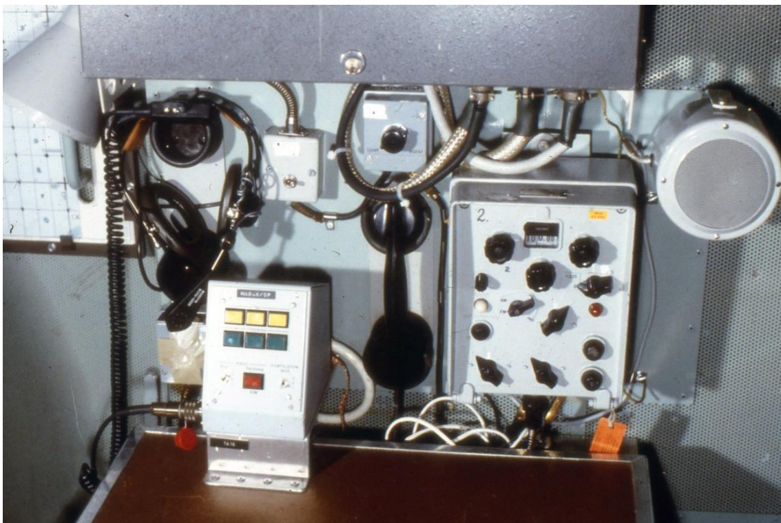
42. Rbb typ Norrköping. Stridsledningscentral, UK-plats
