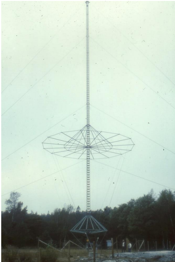
143. Ryssjantenn
