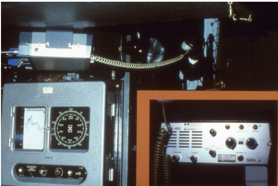
80. Minsvepare typ kust. VHF-station akterut i styrhytt. (VHF-stationen även infälld i bilden)
