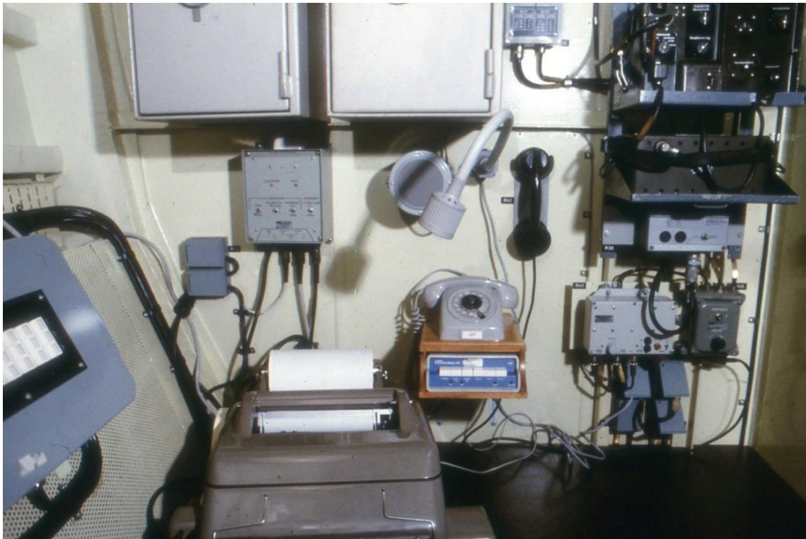
21. Ptrb typ Hugin. Radiohytt, fjärrskrift med modem och Ra 121
