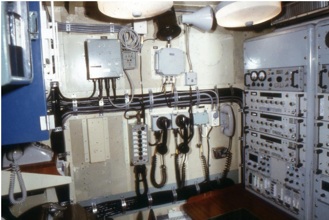
39. Robotbåt typ Norrköping. Radiohytt, betjäningsplats
