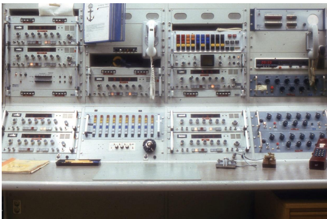
128. Kustradiostation mottagardel. Betjäningsplats A
