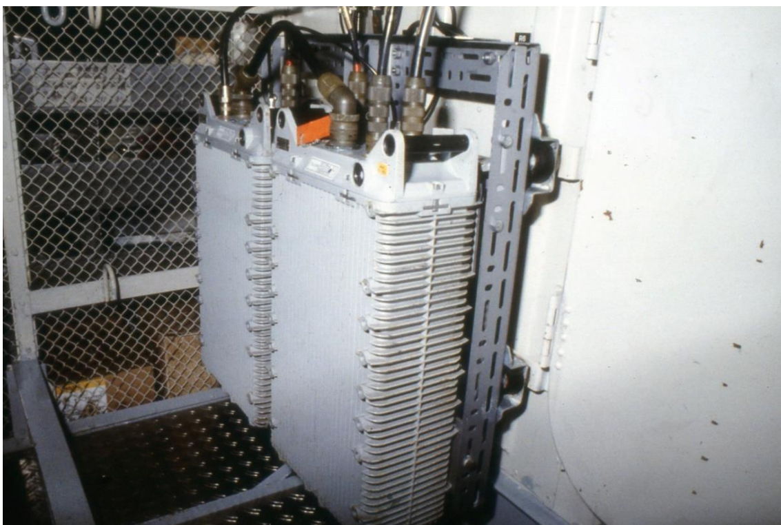
48. Rbb typ Norrköping. RA 800 i gång utanför materielrum
