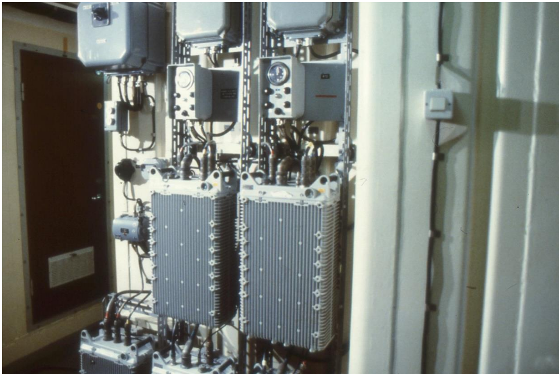
57. Minfartyg typ Älvsborg. RA 800 i gång utanför radiohytt A
