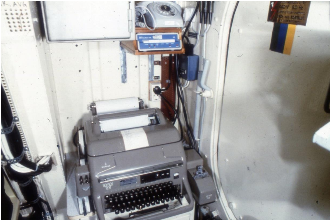
29. Tb typ Spica. Radiohytt, fjärrskrift med modem
