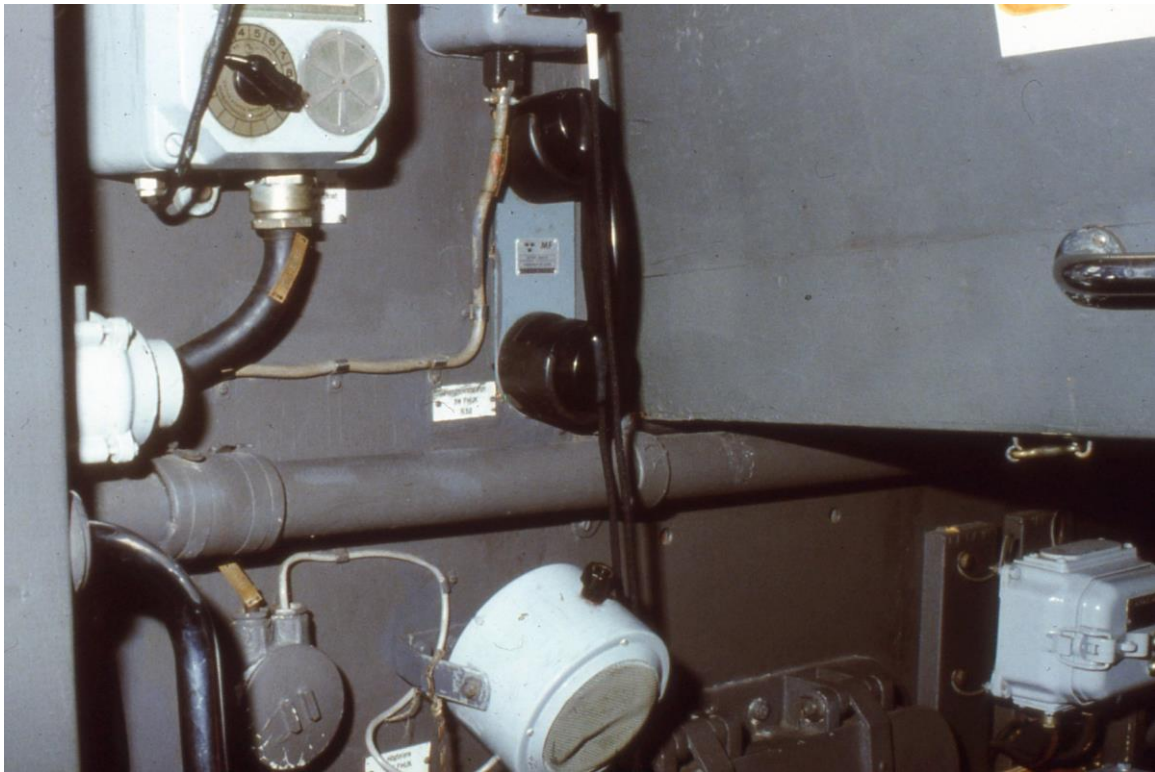
7. Ub typ Sjöormen. Tornet, interiör
