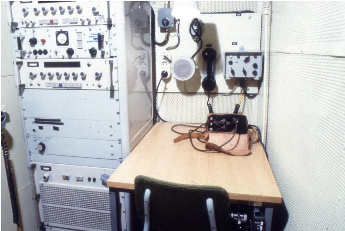
55. Minfartyg typ Älvsborg. Radiohytt B
