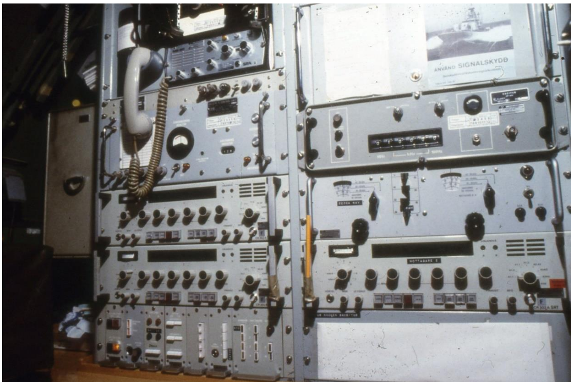
14. ub typ Näcken. Radiohytt, betjäningsplats
