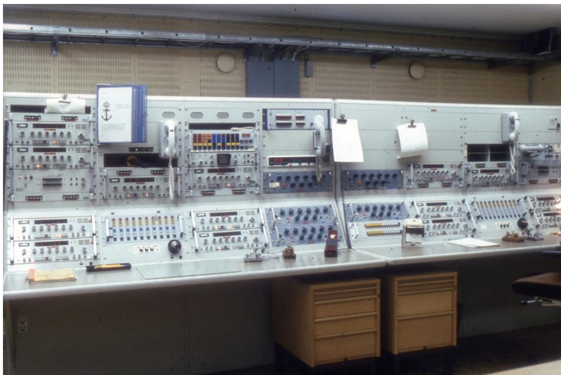
127. Kustradiostation mottagardel. Betjäningsplats för kortvåg
