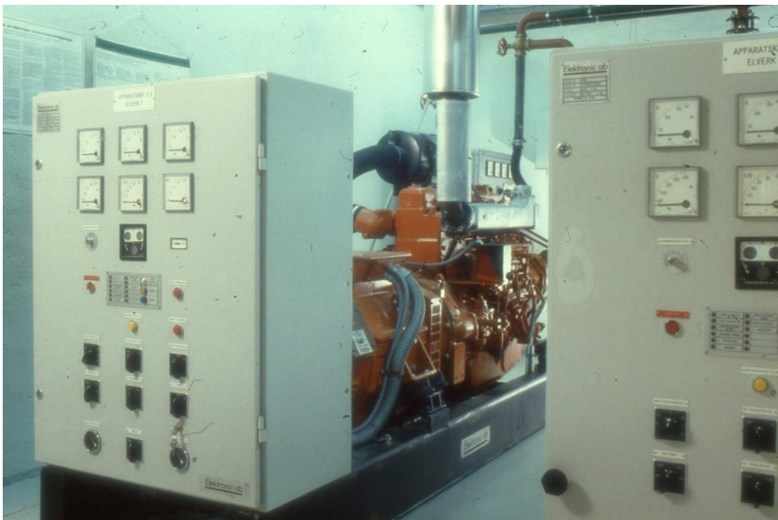
142. Kustradiostation sändardel. Reservkraftaggregat
