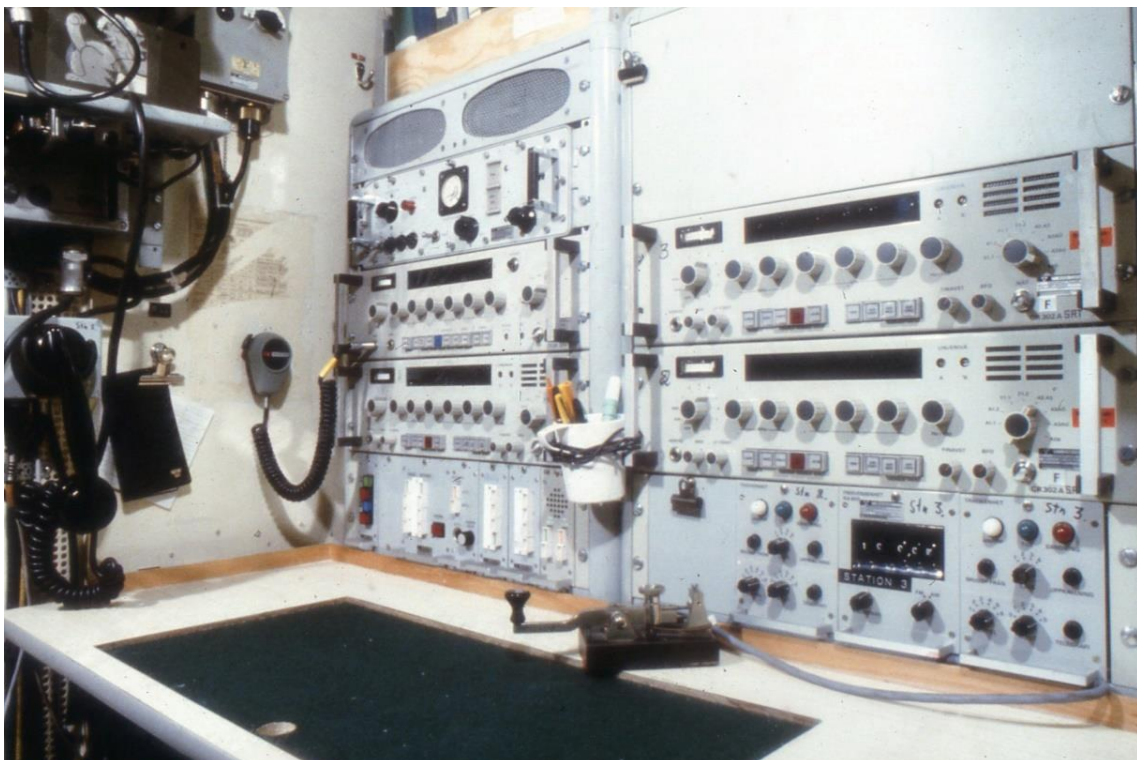
28. Tb typ Spica. Radiohytt, betjäningsplats
