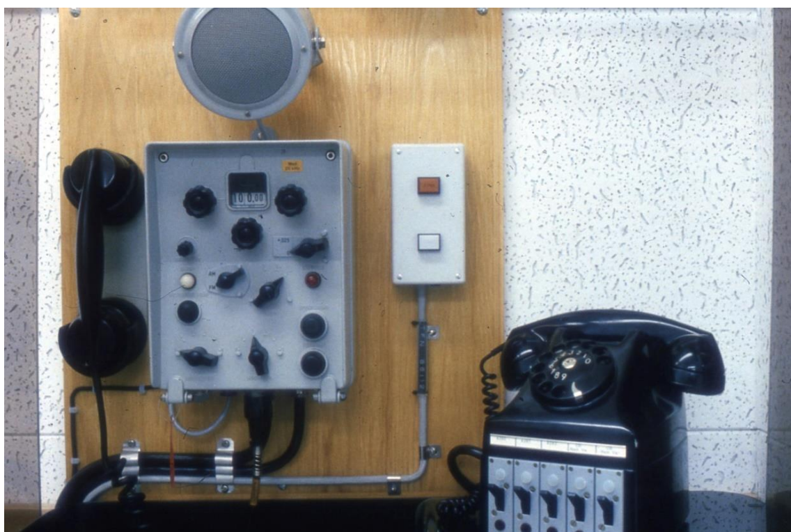
126. Sambandscentral. Radiodetalj, RA 800
