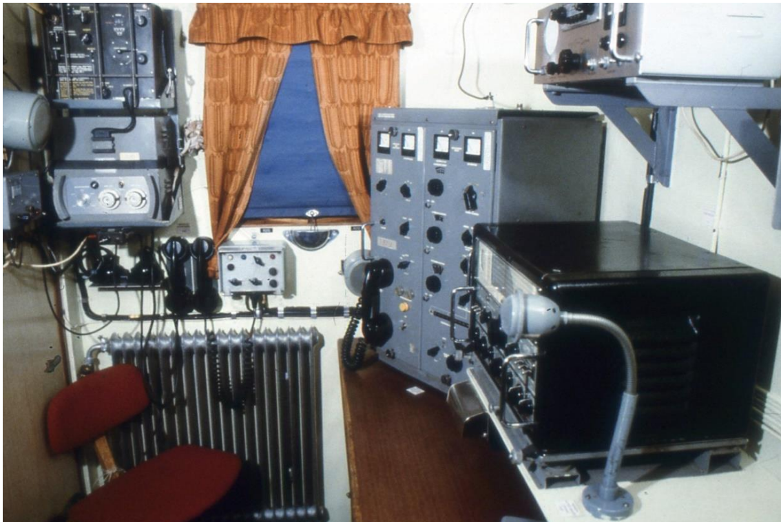
97. Trängfartyg, bogserbåt. Ajax, radiohytt
