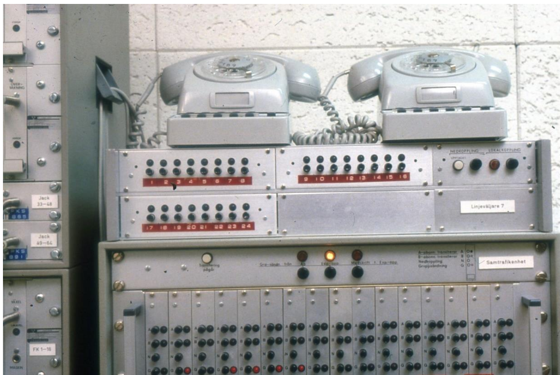
121. Sambandscentral. Linjeväljare
