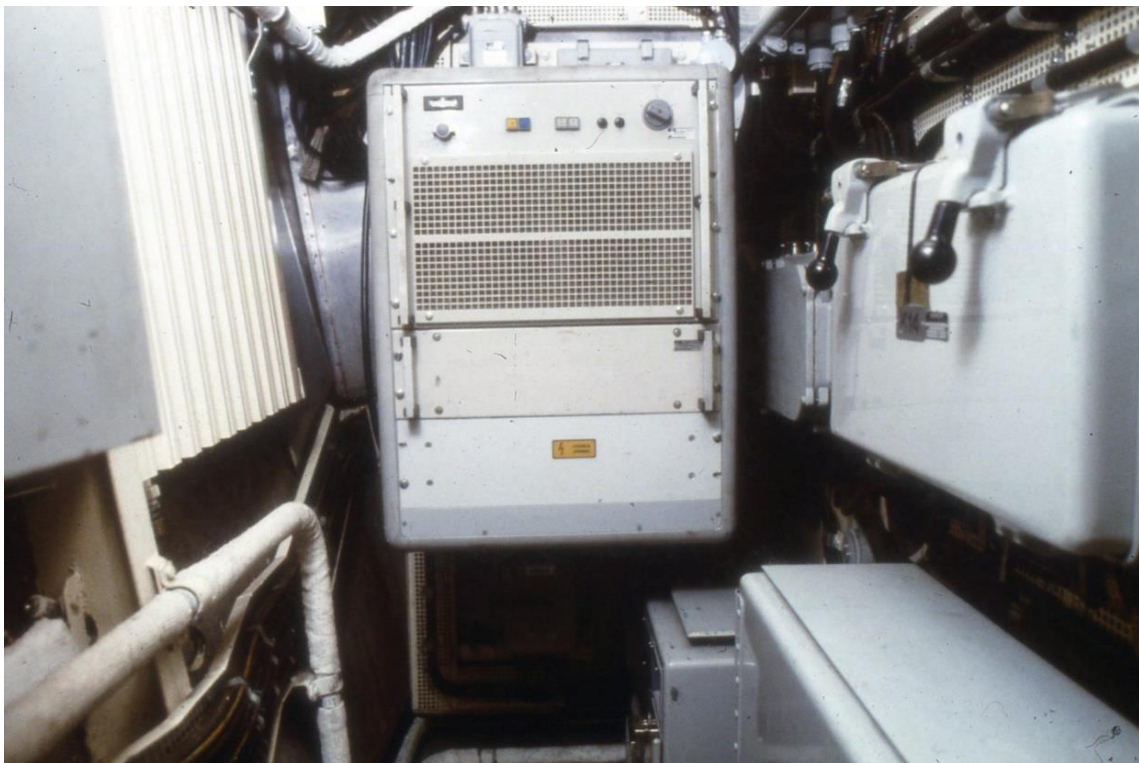
34. Tb typ Spica. Sä 844 i bb apparatrum
