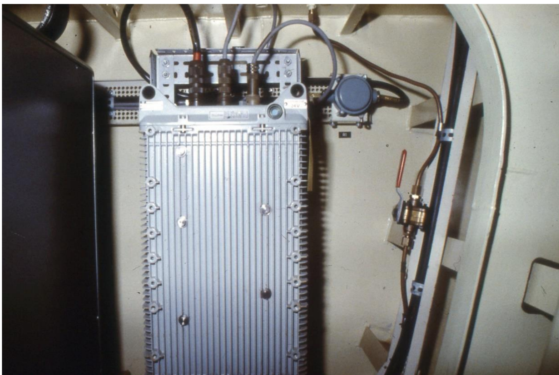
47. Rbb typ Norrköping. RA 800 i elapparaturum under stridsledningscentral
