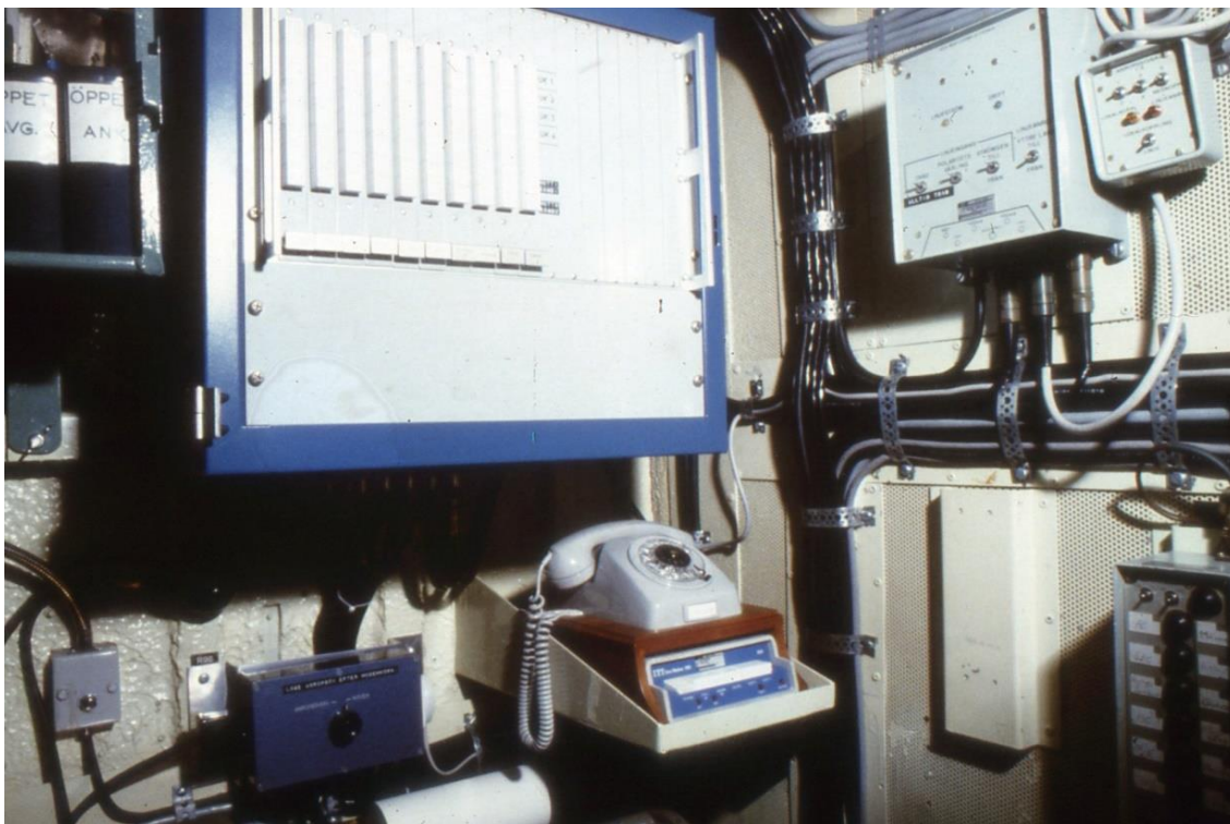
40. Rbb typ Norrköping. Radiohytt, UK-växel och fjärrskriftsutrustning
