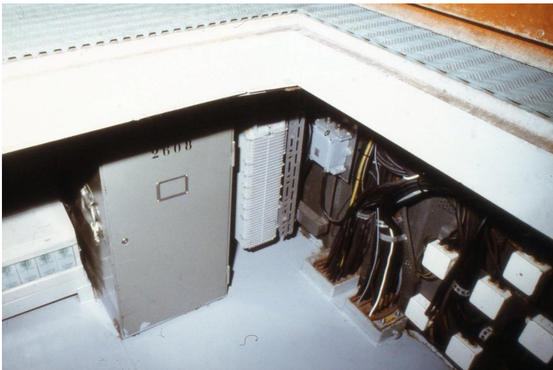
92. Trängfartyg, bärgare. RA 800 i utrymme under styrhytt
