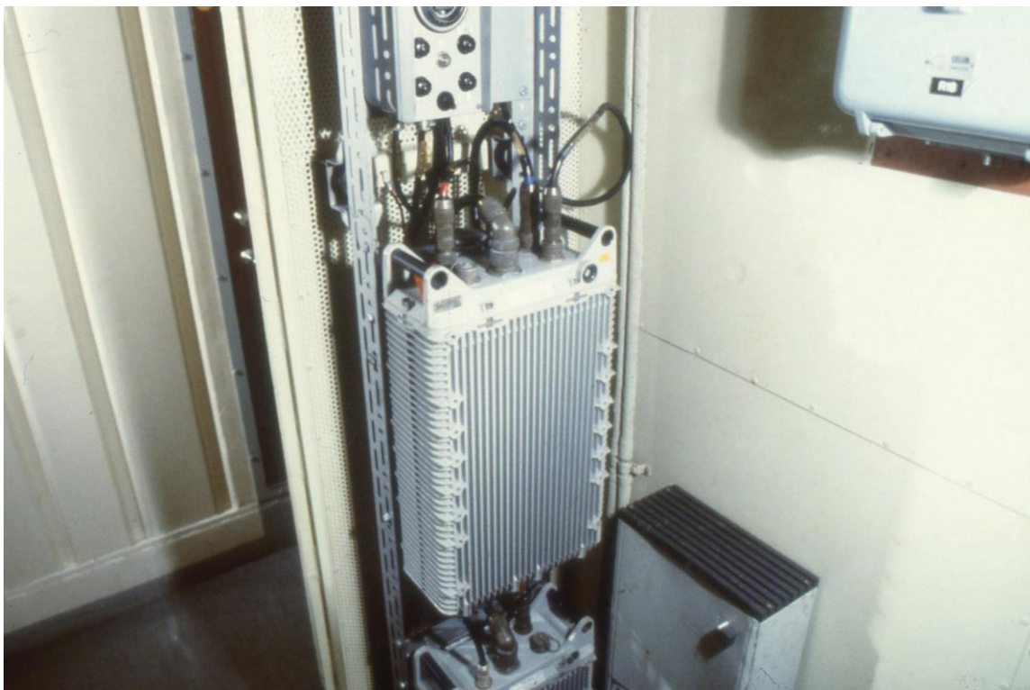
58. Minfartyg typ Älvsborg. RA800 i gång utanför radiohytt A
