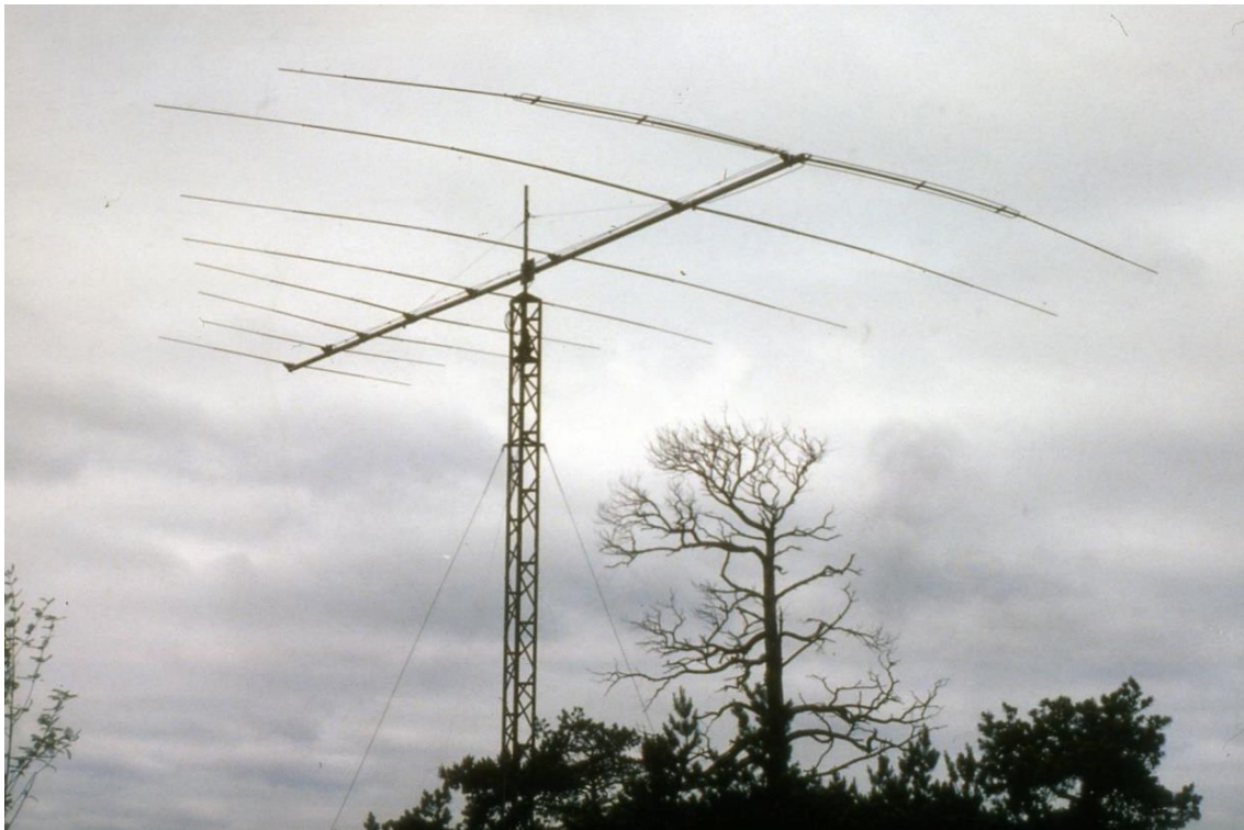
135. Kustradiostation mottagardel. Riktbar kortvågsantenn
