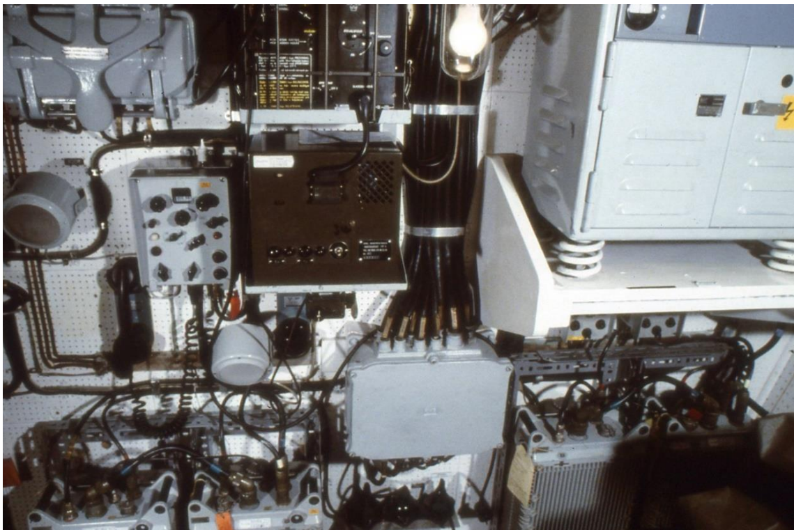
82. Minsvepare typ kust. Radiohytt, RA 800 och RA 121
