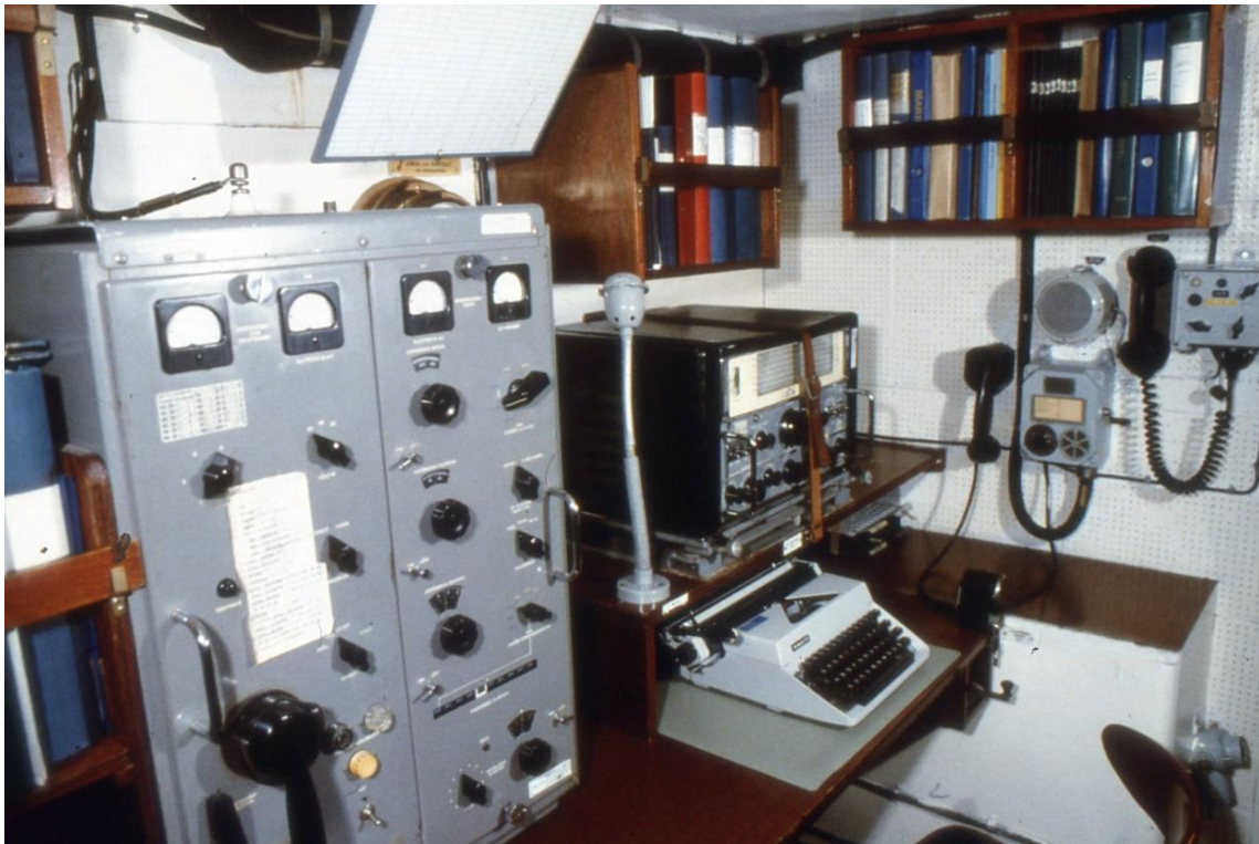
81. Minsvepare typ kust. Radiohytt, betjäningsplats
