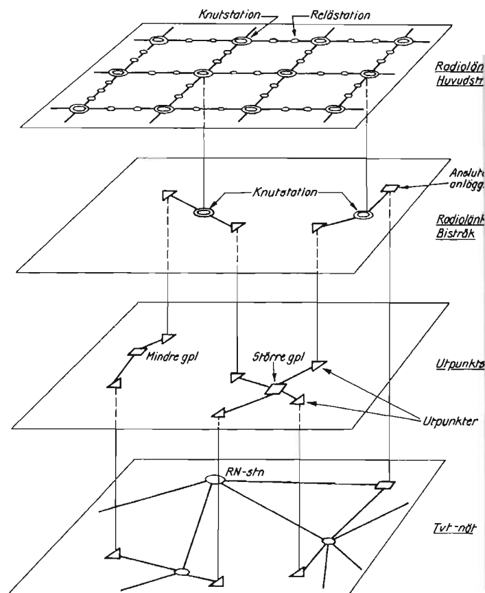
Anläggningars anslutning till olika transmissionsnät
