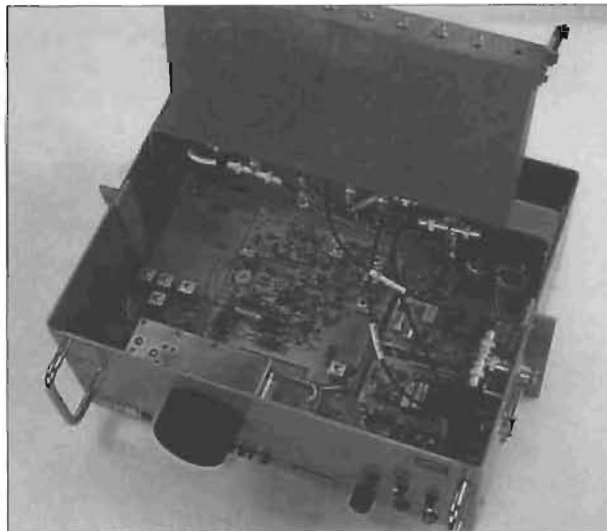
RL-23 (SRA)
