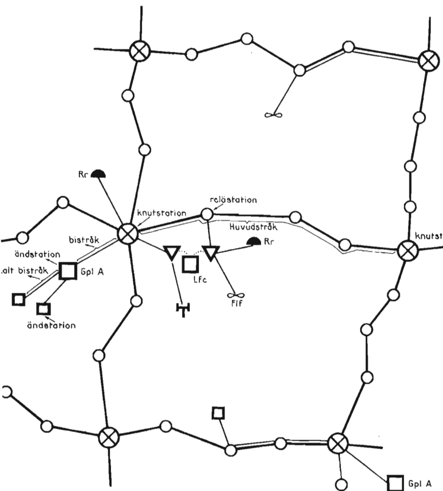
FFRL principiell nätbild
