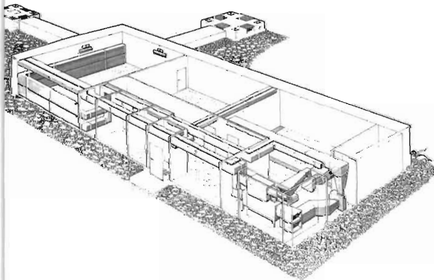
Standardbunker för länkanläggning i FFRL stomdel
