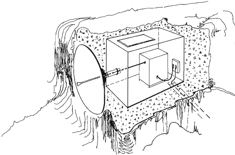
Hårdgjord länkterminal
