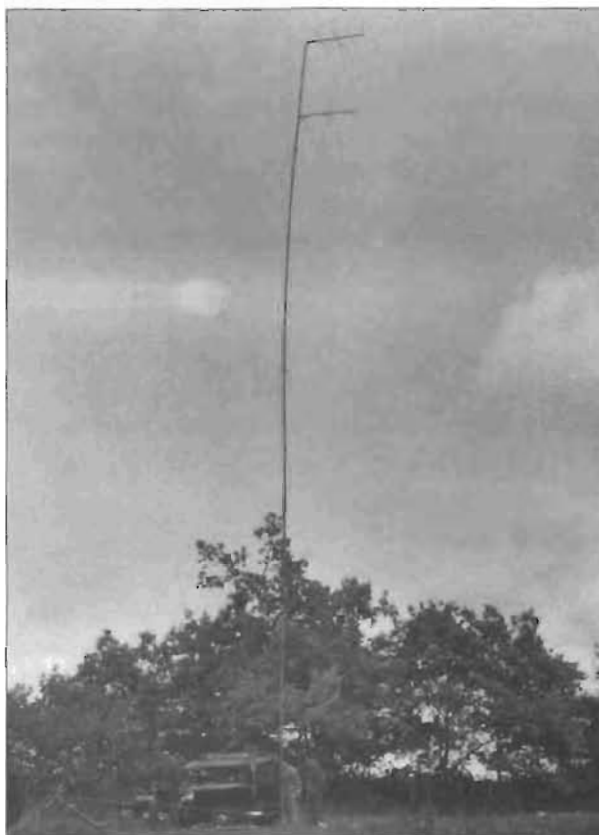
Fältstyrkemätning för RL-02 förbindelse, mast med två yagi-antennor.
