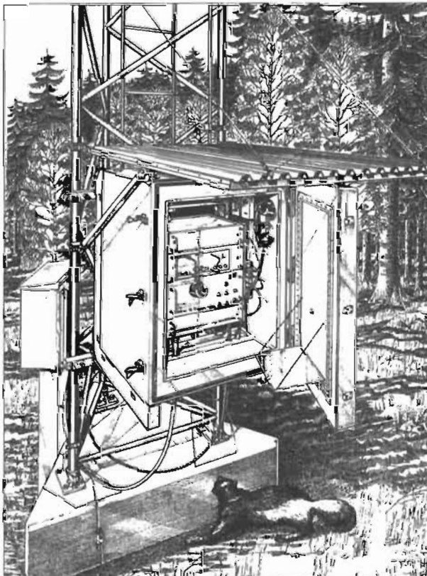
Skåp för fältförbands anslutning till fasta länknätet
