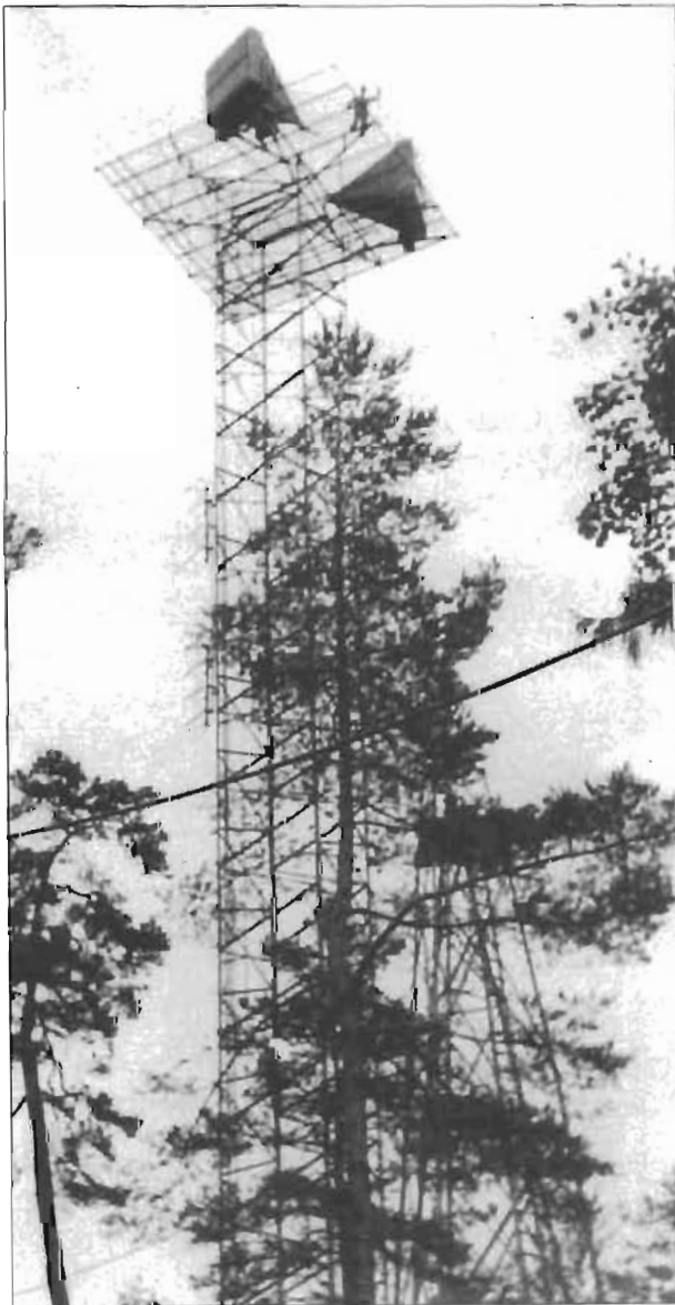
Antenntorn med två Siemens linsantenner
