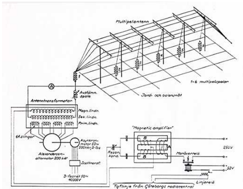
SAQ "blockschema" (Telegrafverkets handbok)
