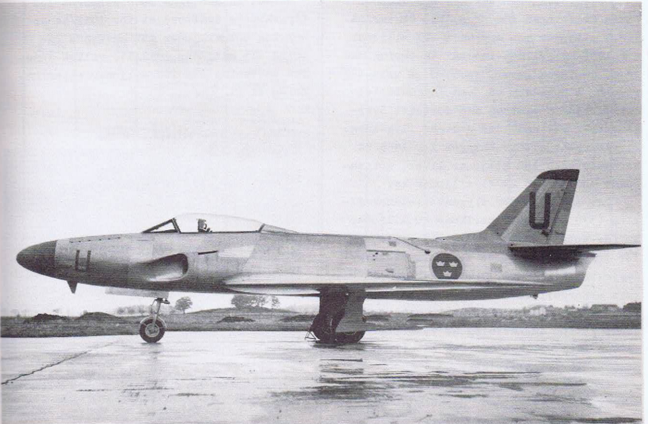
A 32 "Lansen". Besättningen placerad i tandem. Max. hast. över 1.100 km/tim. Motor: en Rolls Royce Avon. Beväpning: automatkanoner, bomber och raketer.
