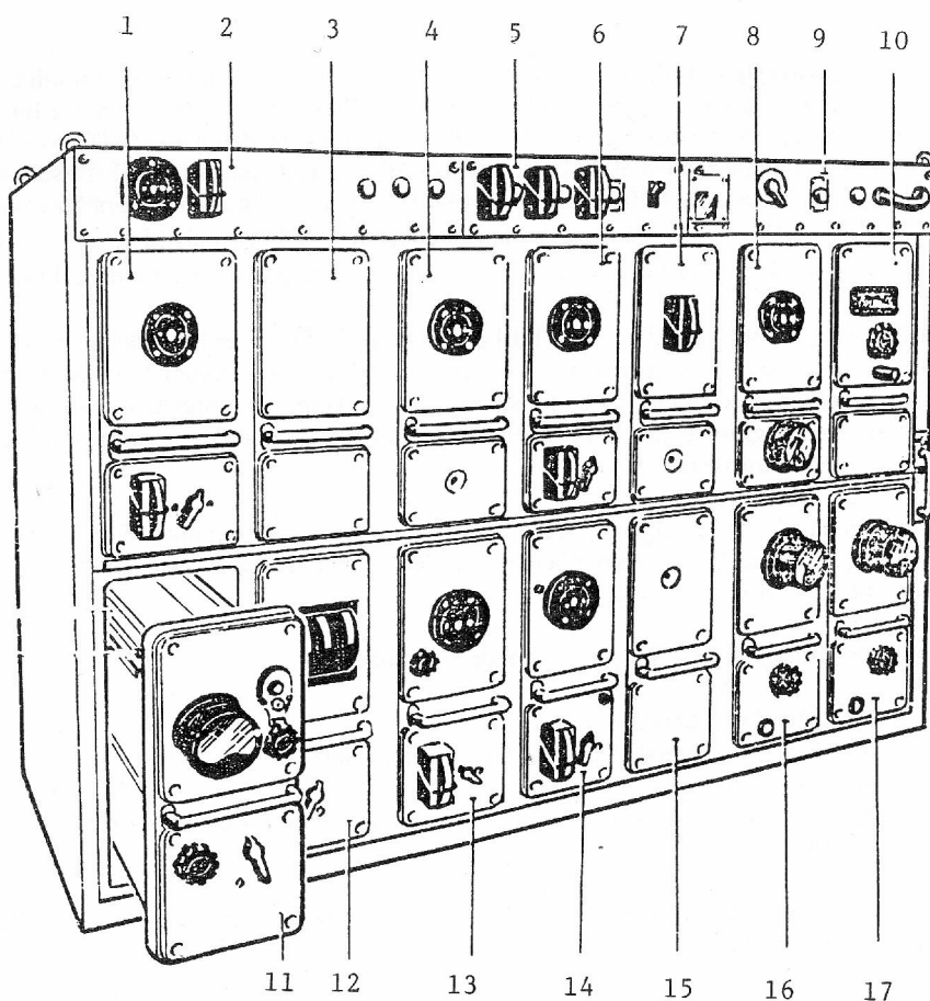
Bild 1. Mottagarenhet PS-16
