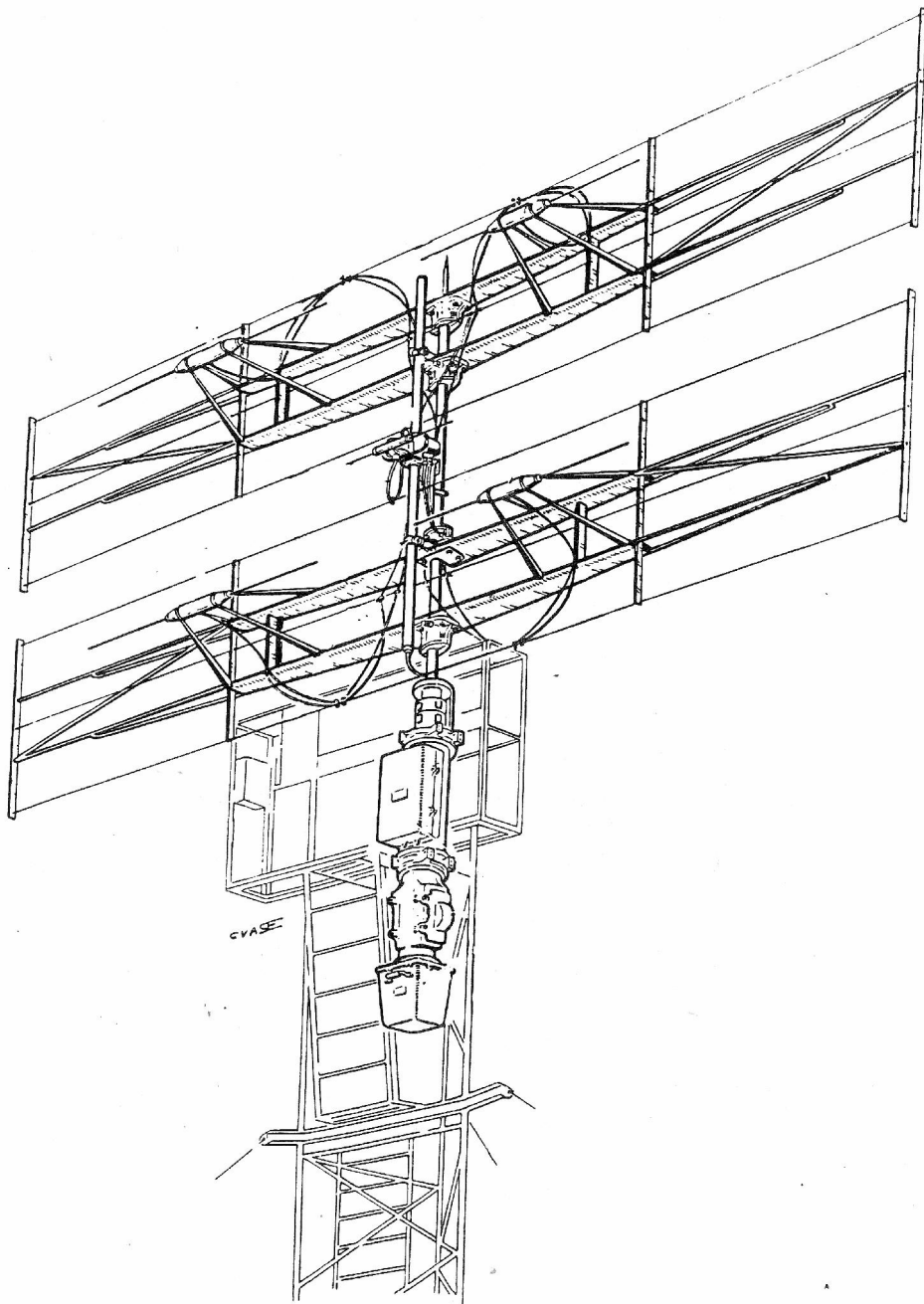
Bild 3. Antenn med antennvridbord PS-16/F
