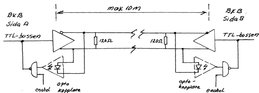
Balanserad transmissionslänk
