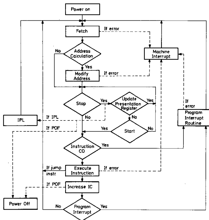
Styrenhetens flödesschema
