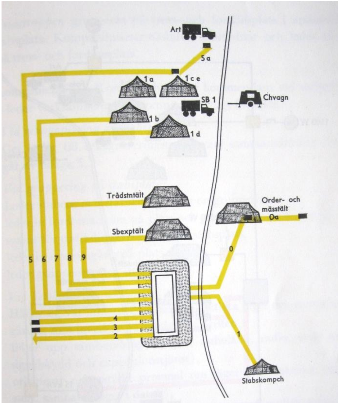
TELE-stomnät Förstabsplats 1
