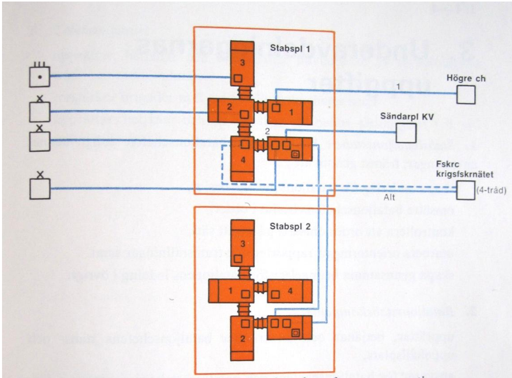
Fjärrskriftsnät Fördelningsstabsbat 73
